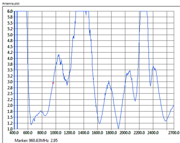
VSWR
